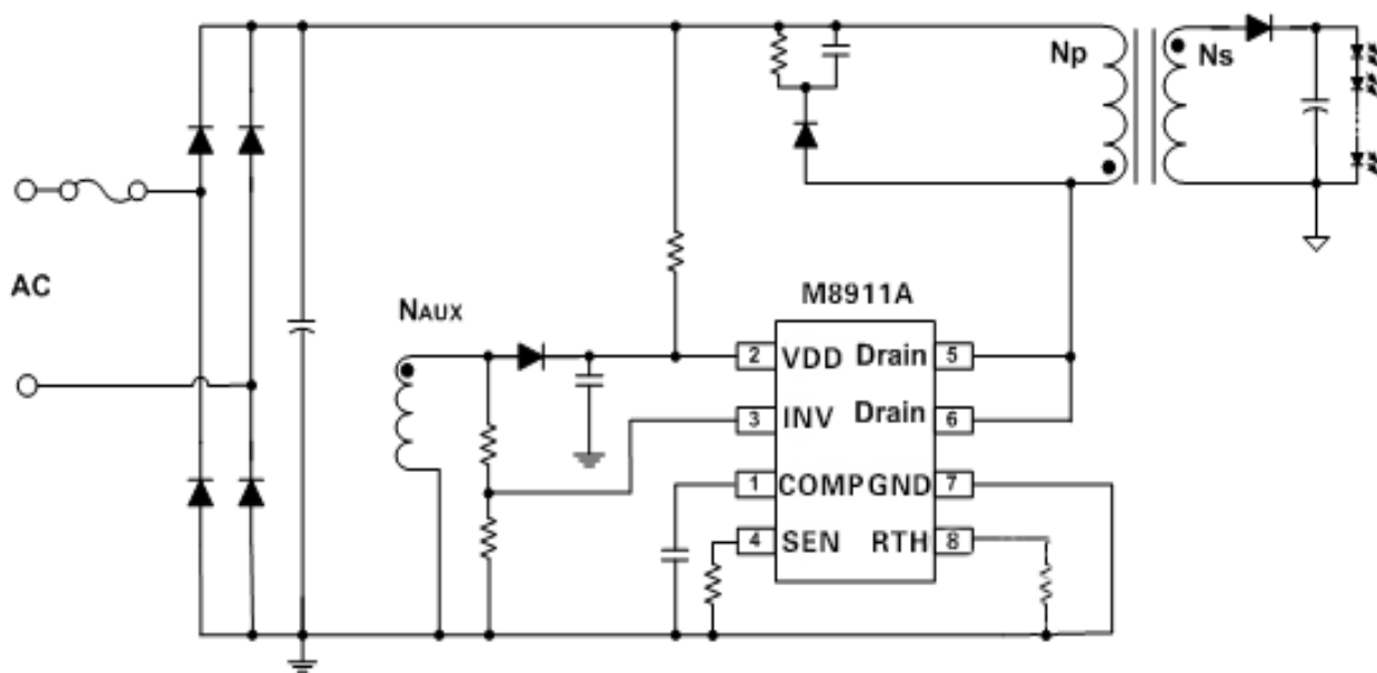
图 1 M8911A 典型应用图
