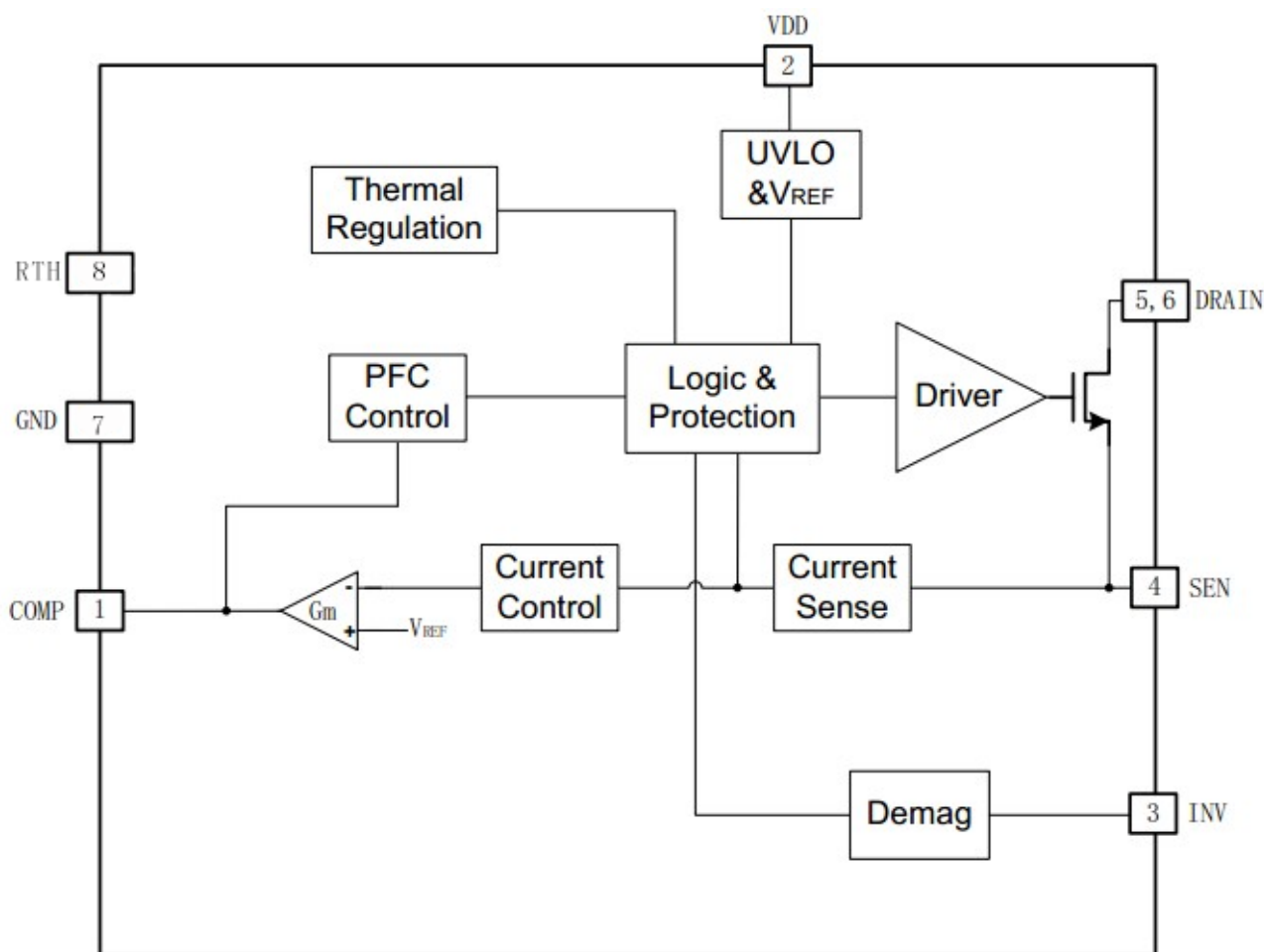
图 3 M8911A 内部框图
