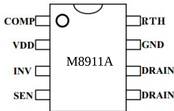
图 2 M8911A 管脚排列图
